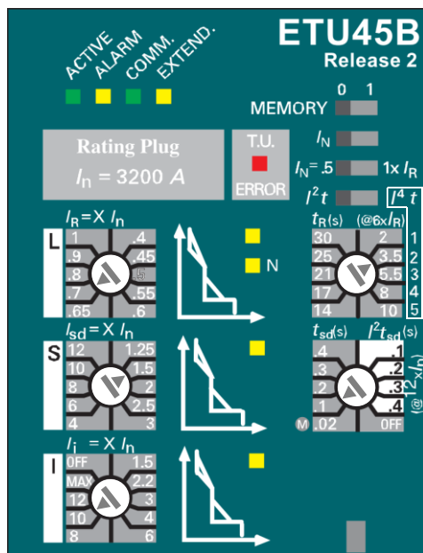
Figuur 31 Siemens ETU45B LSI-relais
