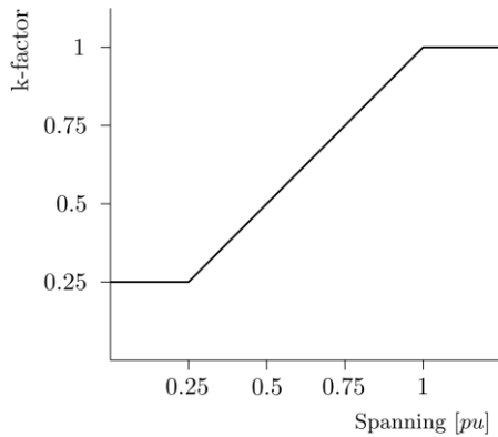
Figuur 10 Spanningsproportionele overstroombeveiliging, k-factor
