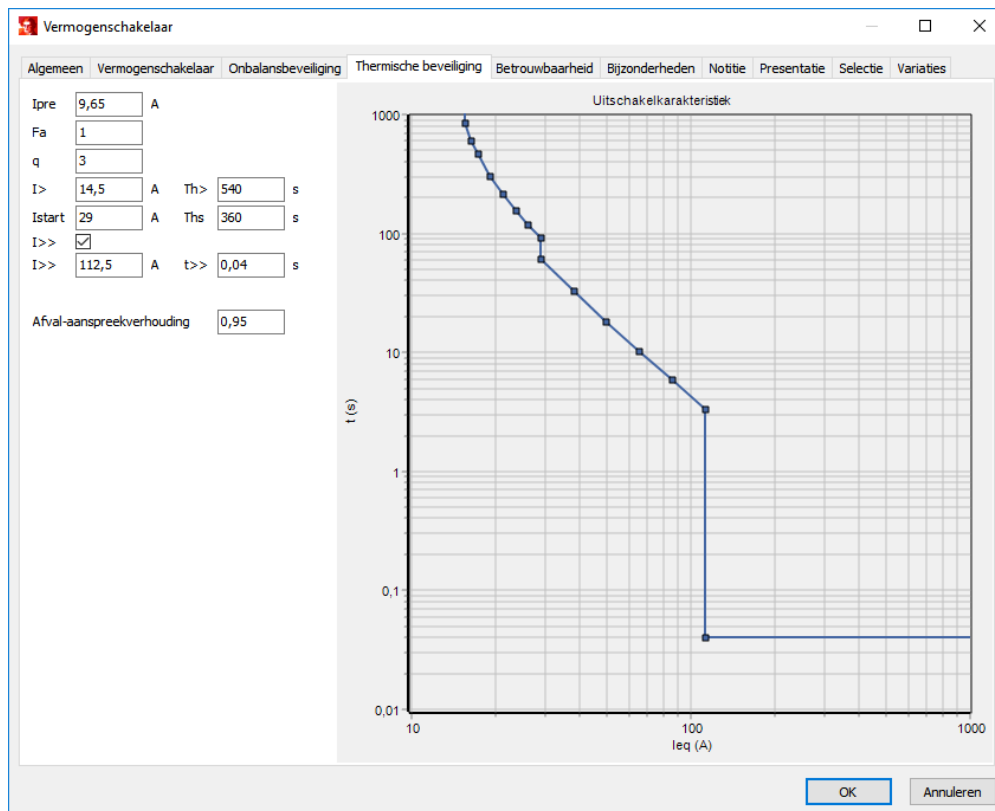
Figuur 29 Invoer thermisch relais Vision Network Analysis
