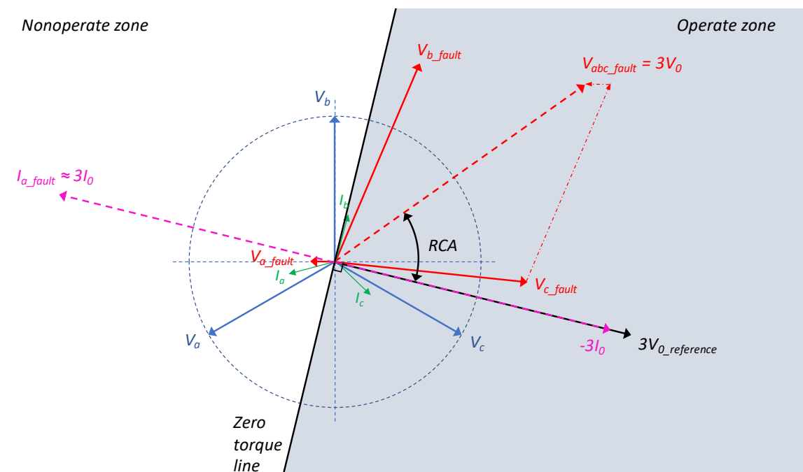
Figuur 23 Vectordiagram energierichtingrelais, aardfout ANSI 67N
