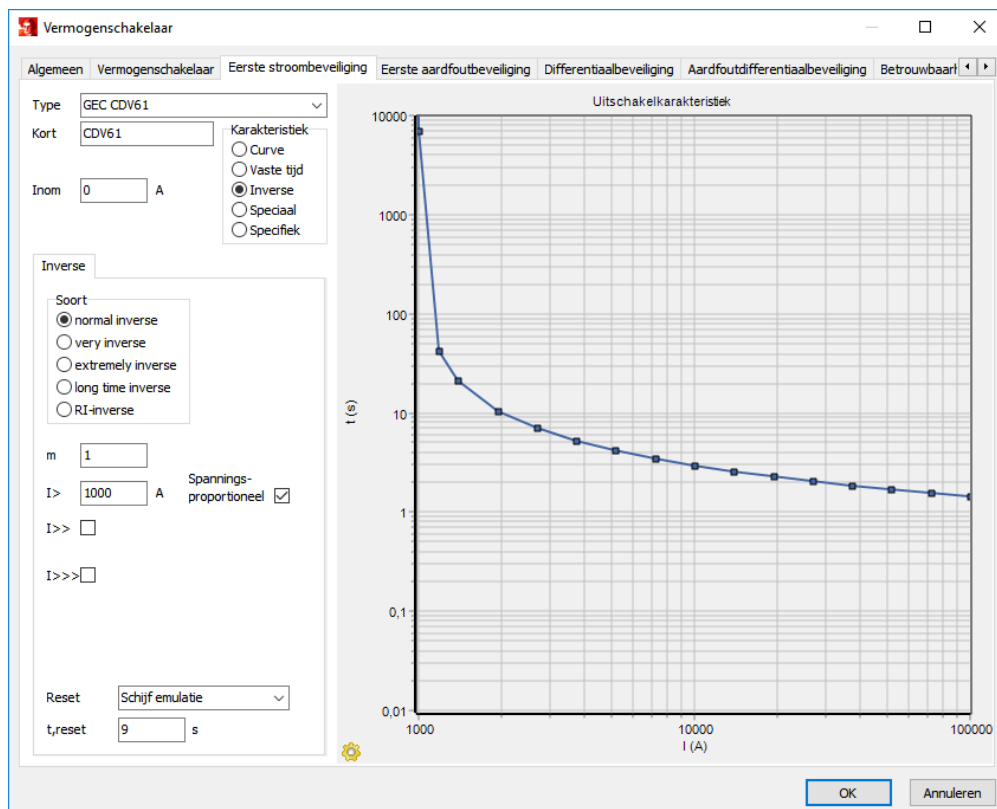
Figuur 12 Implementatie spanningsproportionele overstromfunctie in Vision
