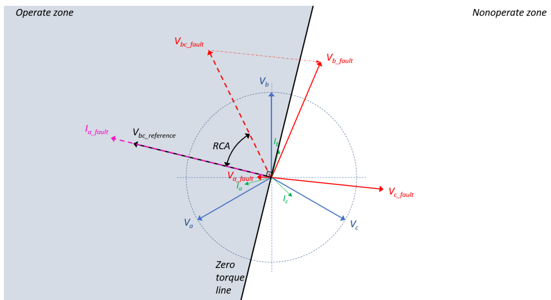
Figuur 25 Vectordiagram energierichtingsrelais, overstroom ANSI 67
