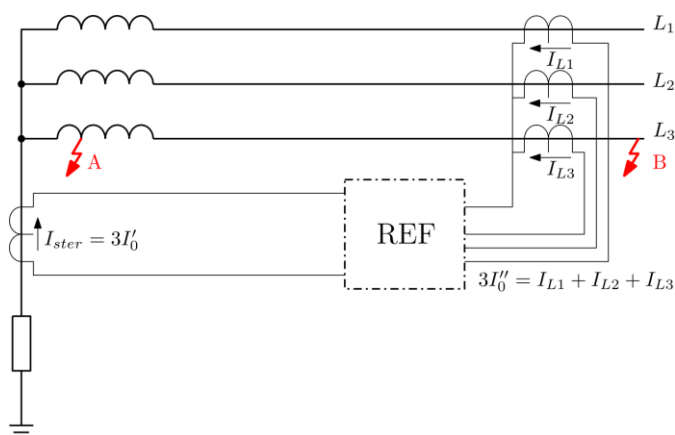
Figuur 26 Aardfoutdifferentiaalbeveiliging principe
