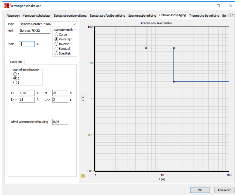
Figuur 28 Invoer onbalansbeveiliging Vision Network Analysis
