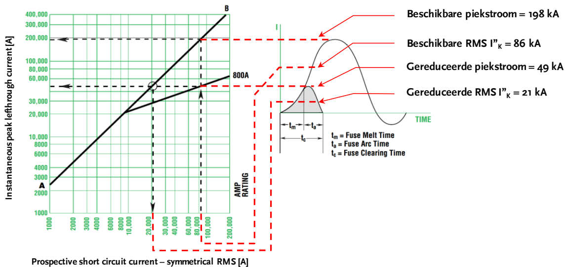
Figuur 21 Kapstroomwerking principe smeltveiligheid
