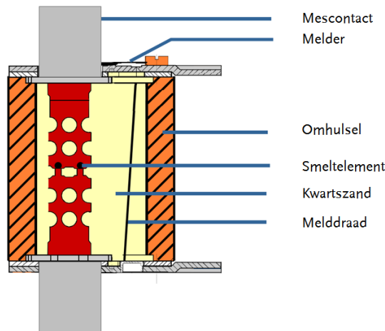
Figuur 18 Mespatroon (Bron: ZVEI)
