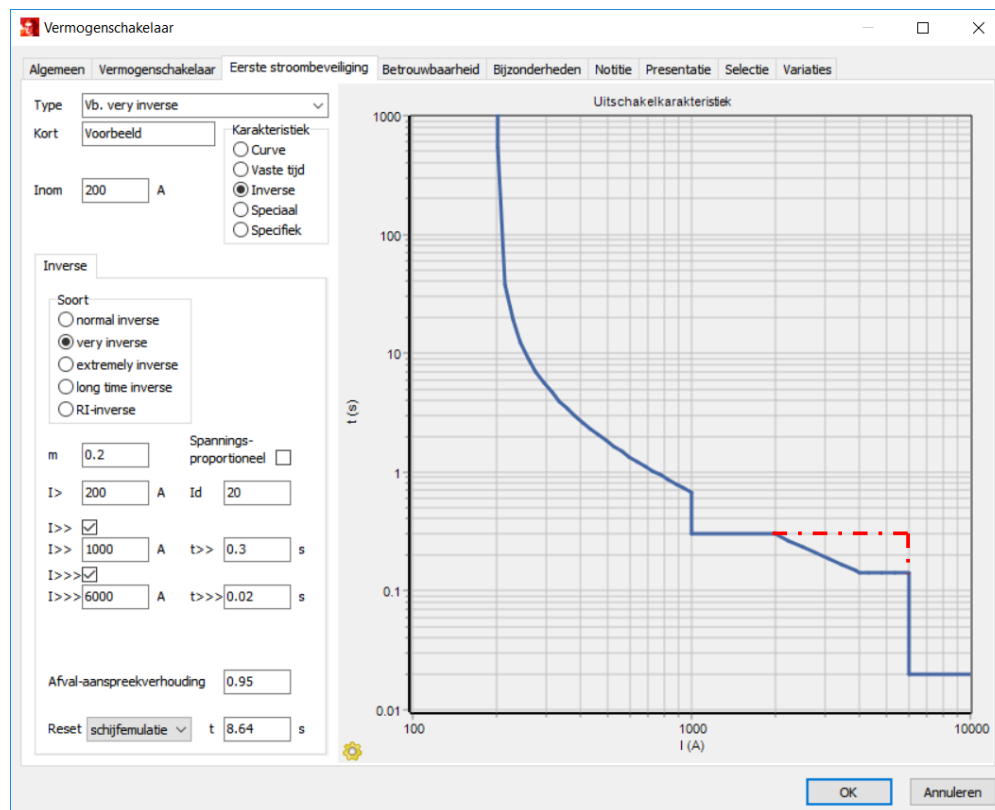
Figuur 8 Invoer overstroomrelais met meerdere trappen
