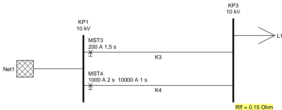
Figuur 15 Netwerk voorbeeld 3 Vision Network Analysis
