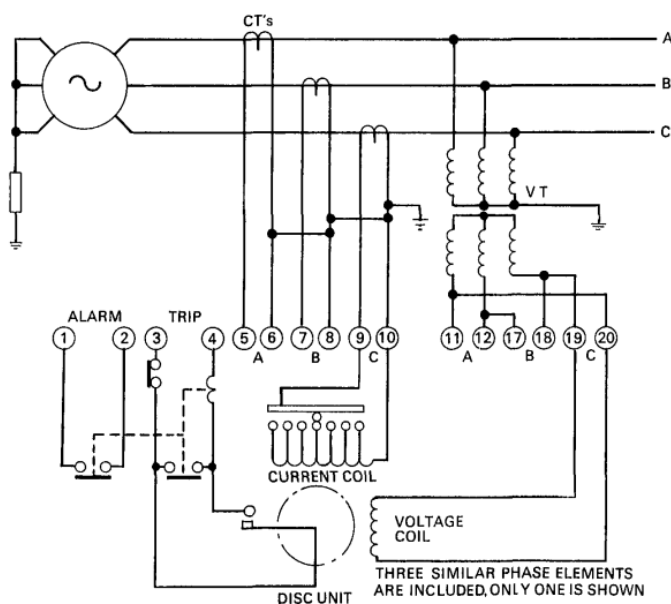
Figuur 9 Spanningsproportioneel overstroombestanddeel GEC CDV61 (GEC)
