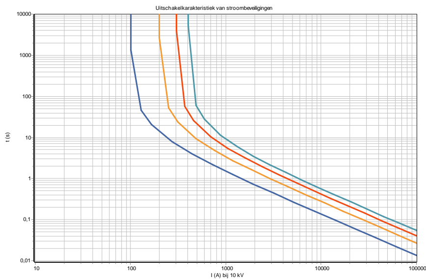
Figuur 11 Inverse overstromkarakteristiek bij verschillende spanningniveaus
