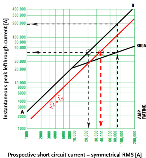
Figuur 22 Kapstroomwerking bij kappa gelijk aan 1
